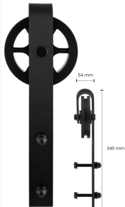
Schuifdeurhanger Teho Per stuk, twee nodig per deur
