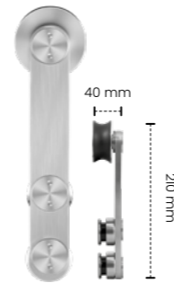
Schuifdeurhanger Linja Per stuk, t.b.v. glasdeuren
