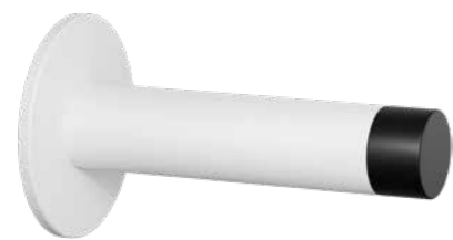
GPF8736 62 000 ∅ 19/50 | ↔ 85
